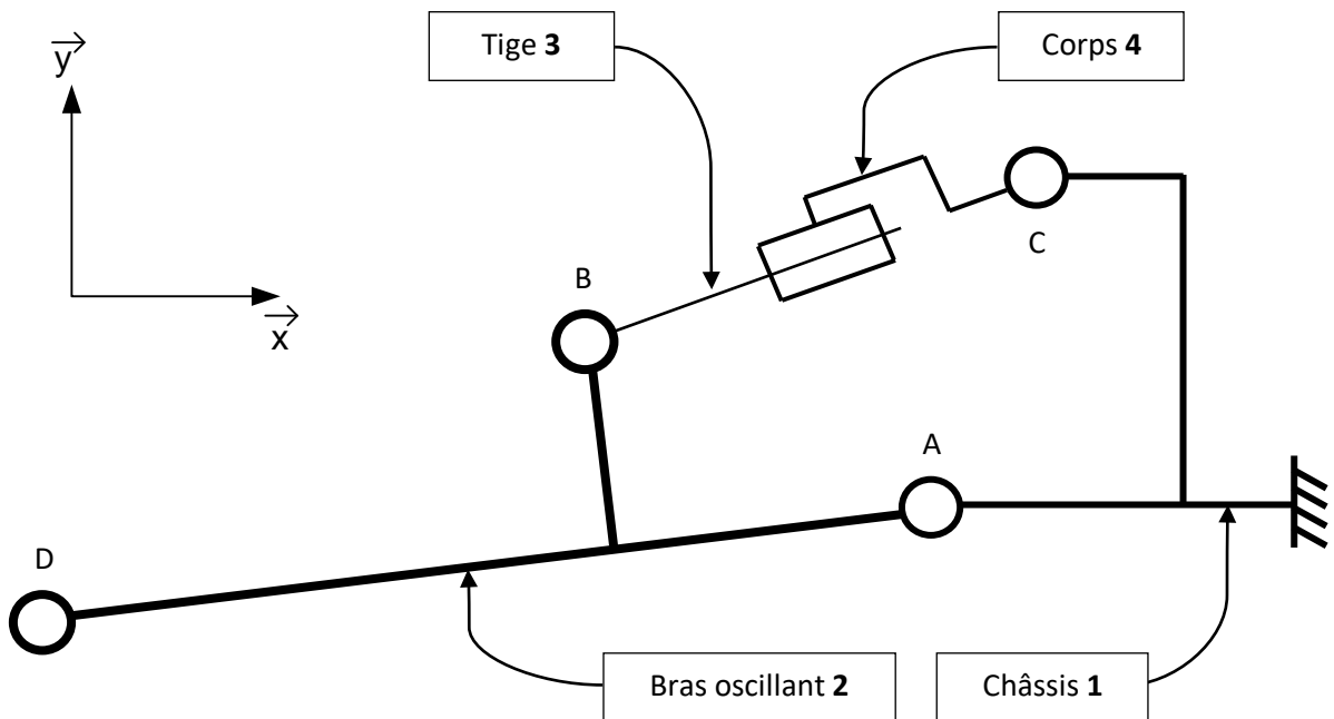
Schéma cinématique de la suspension arrière
