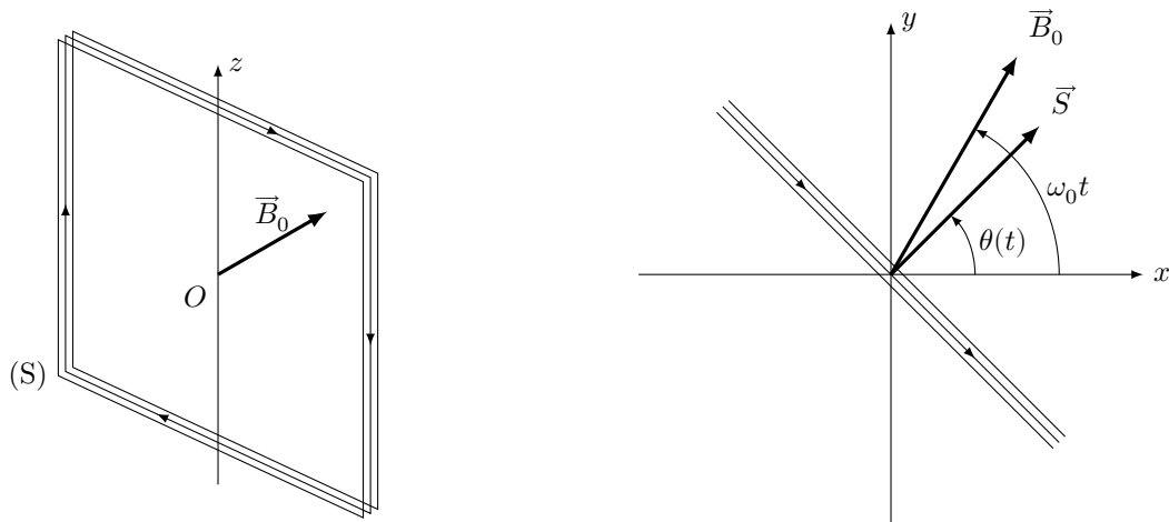
Figure 11 Bobine rectangulaire
