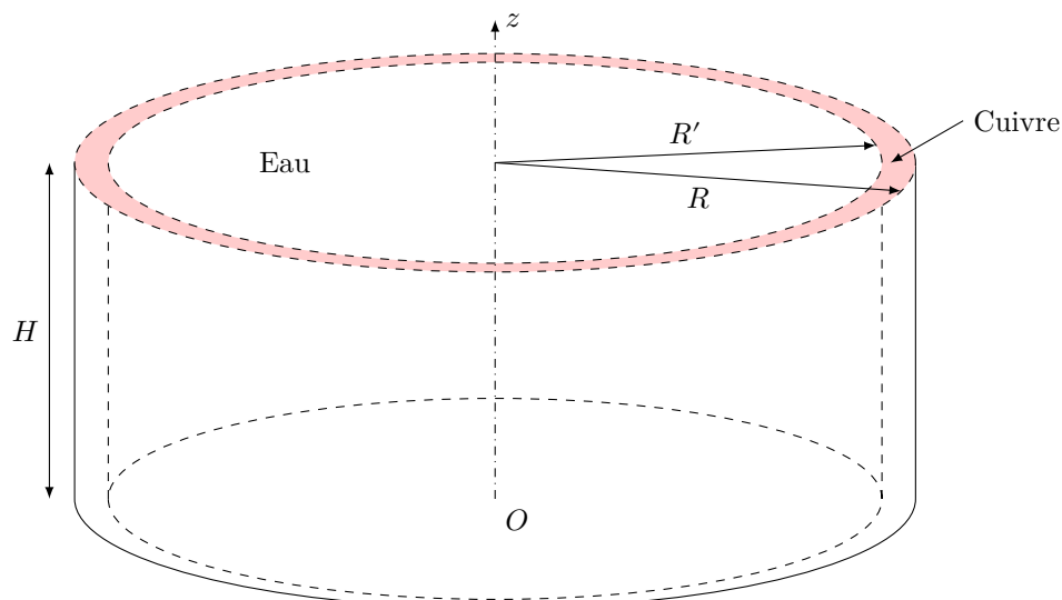
Figure 7 Diffusion thermique
