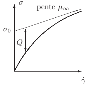
FIG. 32 – Rhéogramme du fluide de Shandraw.
