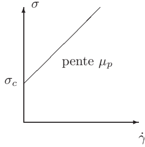
FIG. 27 – Rhéogramme d'un fluide de Bingham.
