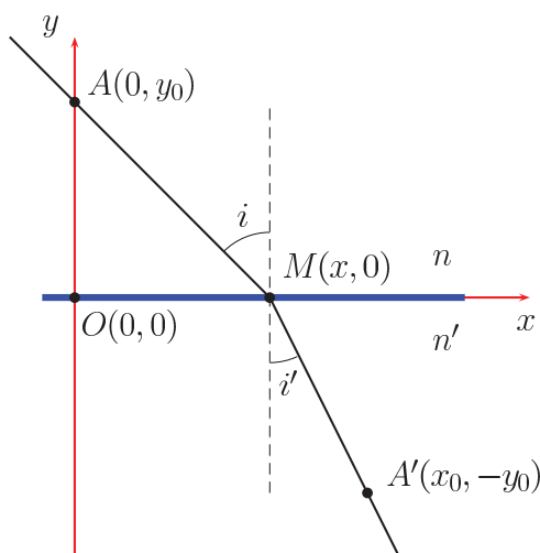
Figure 1. Principe de Fermat et dioptré plan.
