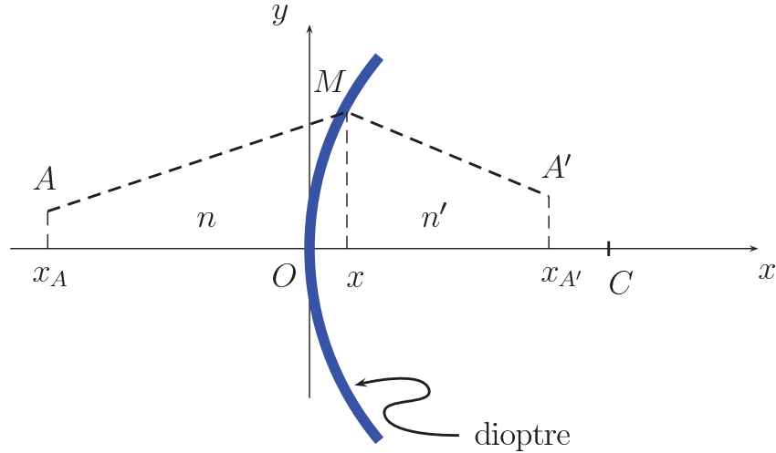
Figure 2. Dioptre sphérique de centre C séparant deux milieux d'indices n et n' .
