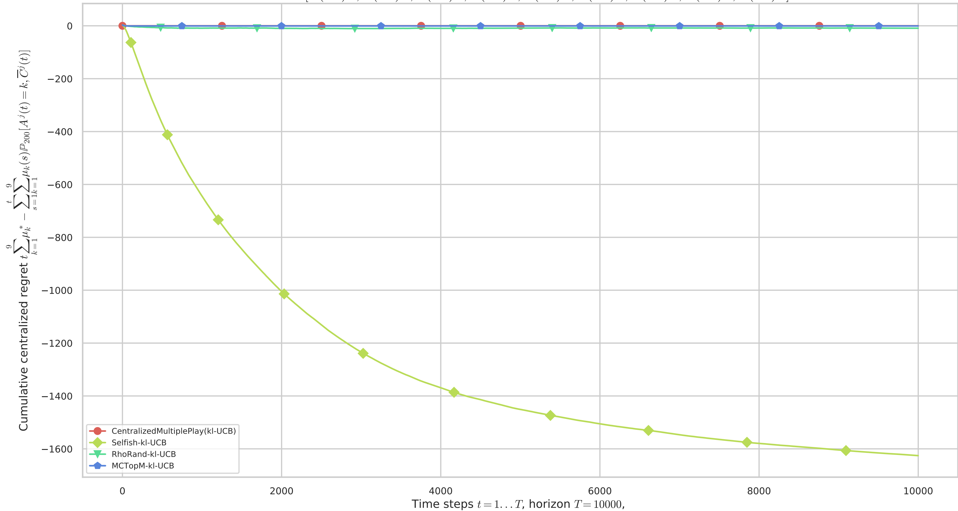
Multi-players M=9 : Cumulated centralized regret, averaged 200 times 9 arms: [B(0.1)^*, B(0.2)^*, B(0.3)^*, B(0.4)^*, B(0.5)^*, B(0.6)^*, B(0.7)^*, B(0.8)^*, B(0.9)^*]
