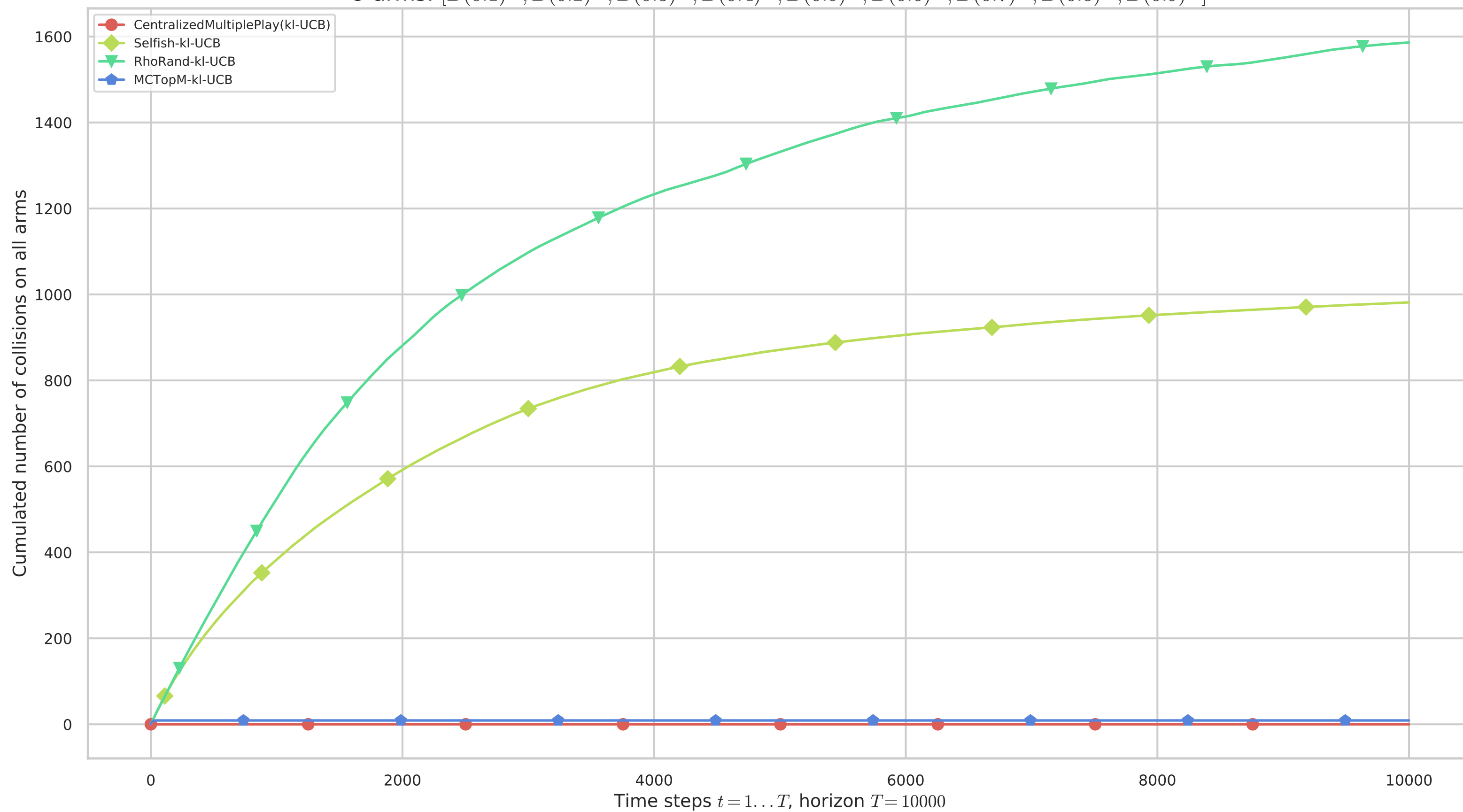
Multi-players M=9 : Cumulated number of collisions, averaged 200 times 9 arms: [B(0.1)^*, B(0.2)^*, B(0.3)^*, B(0.4)^*, B(0.5)^*, B(0.6)^*, B(0.7)^*, B(0.8)^*, B(0.9)^*]
