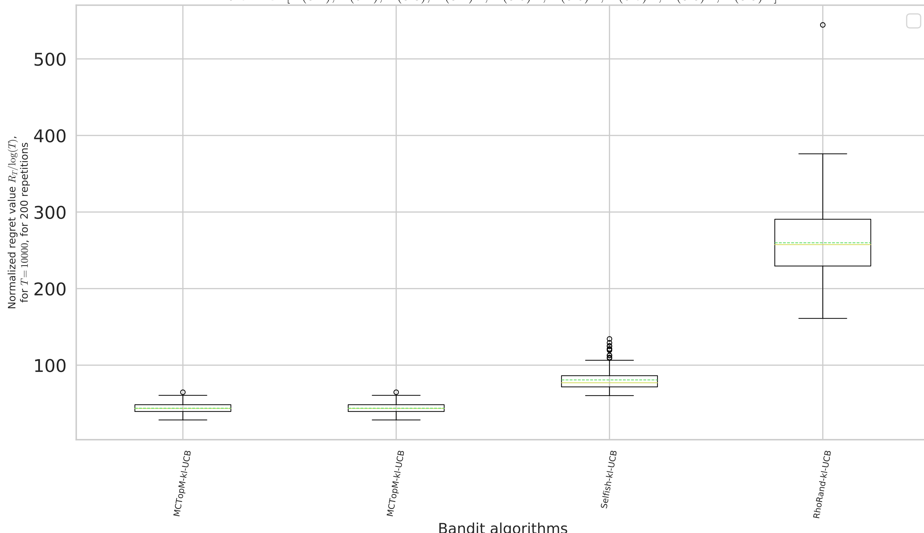
Multi-players M=6 : regrets for different bandit algorithms 9 arms: [B(0.1), B(0.2), B(0.3), B(0.4)^*, B(0.5)^*, B(0.6)^*, B(0.7)^*, B(0.8)^*, B(0.9)^*]
