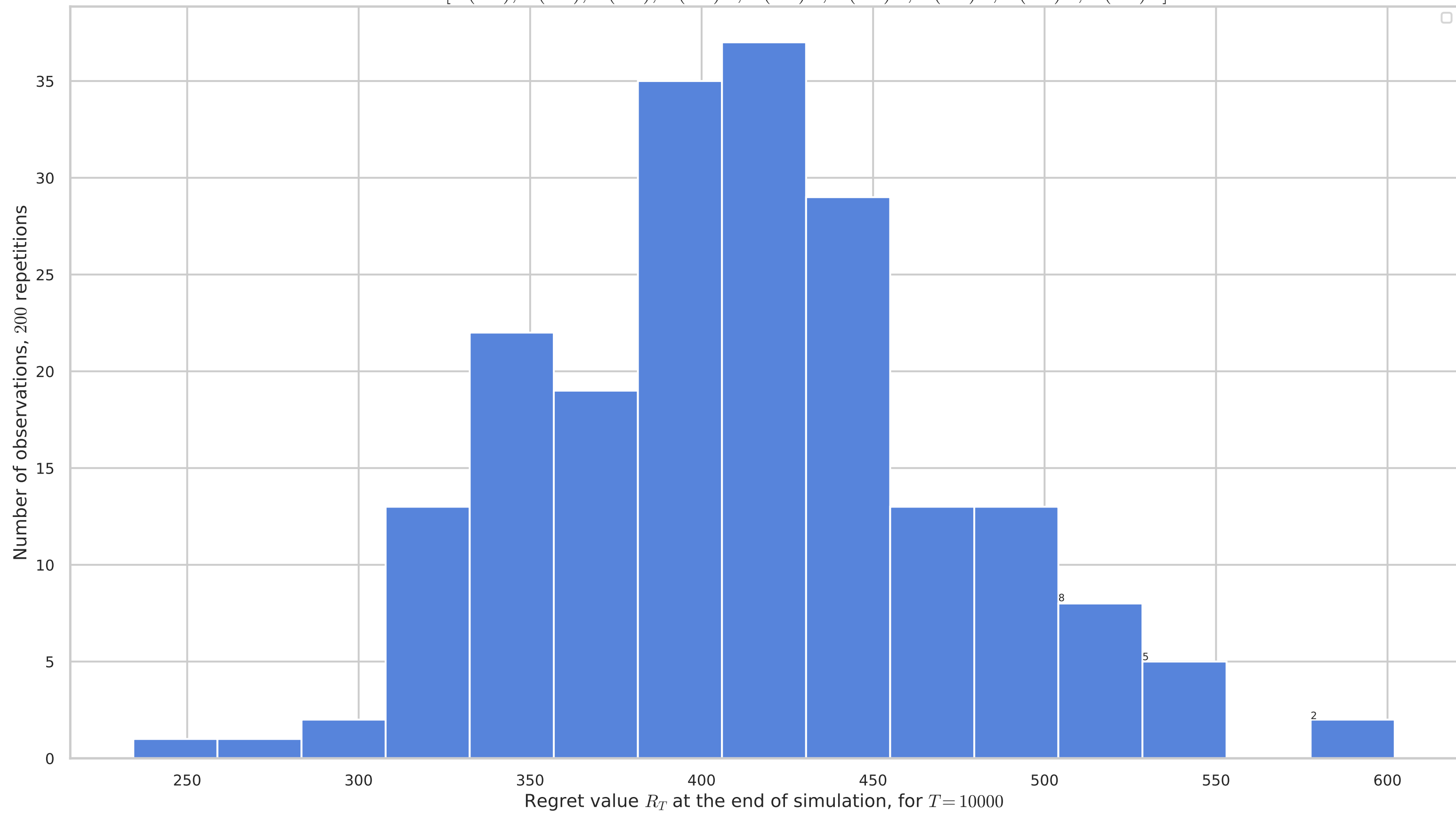
Multi-players M=6 : Histogram of regrets for MCTopM-kl-UCB 9 arms: [B(0.1), B(0.2), B(0.3), B(0.4)^*, B(0.5)^*, B(0.6)^*, B(0.7)^*, B(0.8)^*, B(0.9)^*]
