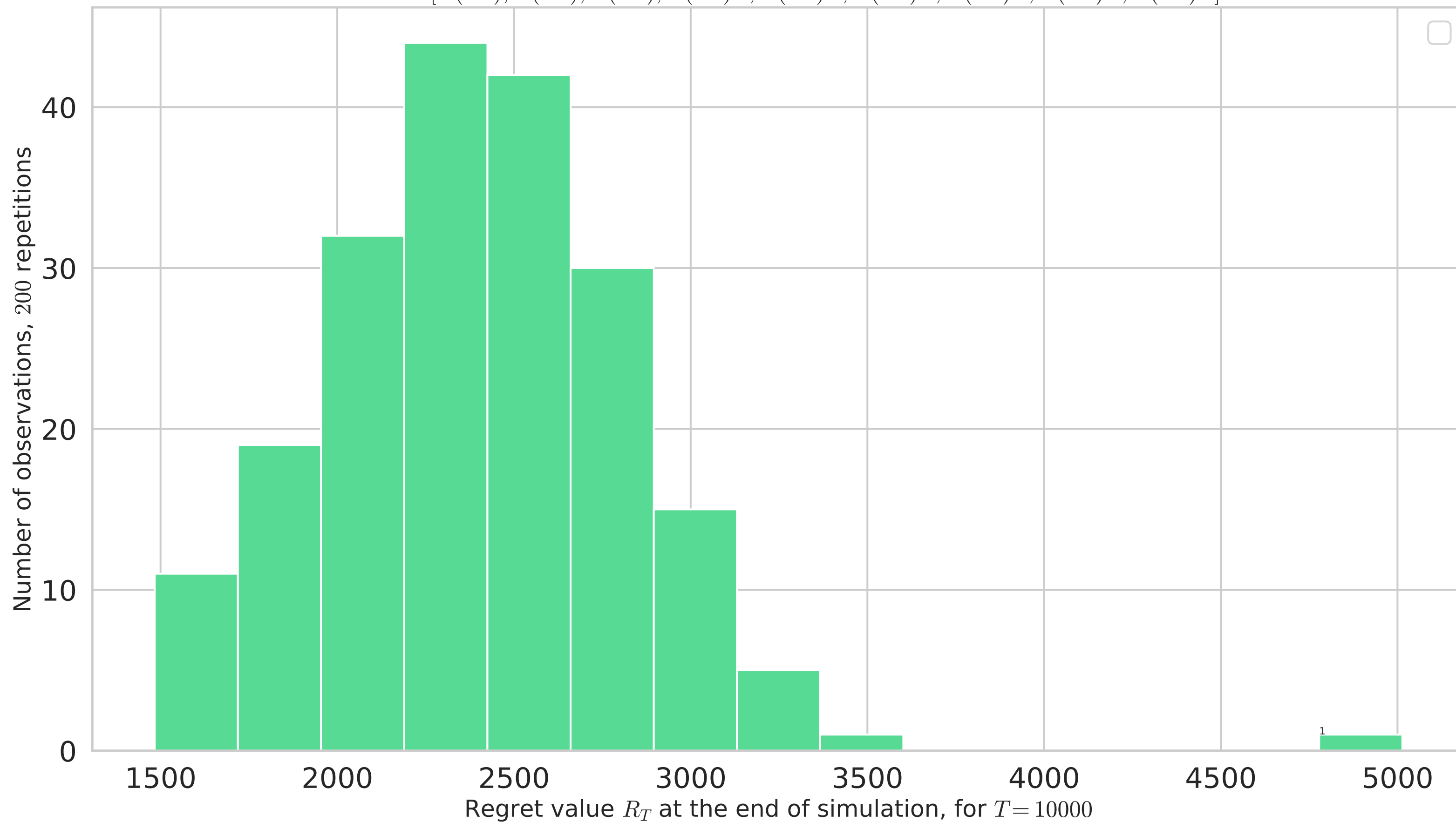
Multi-players M=6 : Histogram of regrets for RhoRand-kl-UCB 9 arms: [B(0.1), B(0.2), B(0.3), B(0.4)^*, B(0.5)^*, B(0.6)^*, B(0.7)^*, B(0.8)^*, B(0.9)^*]
