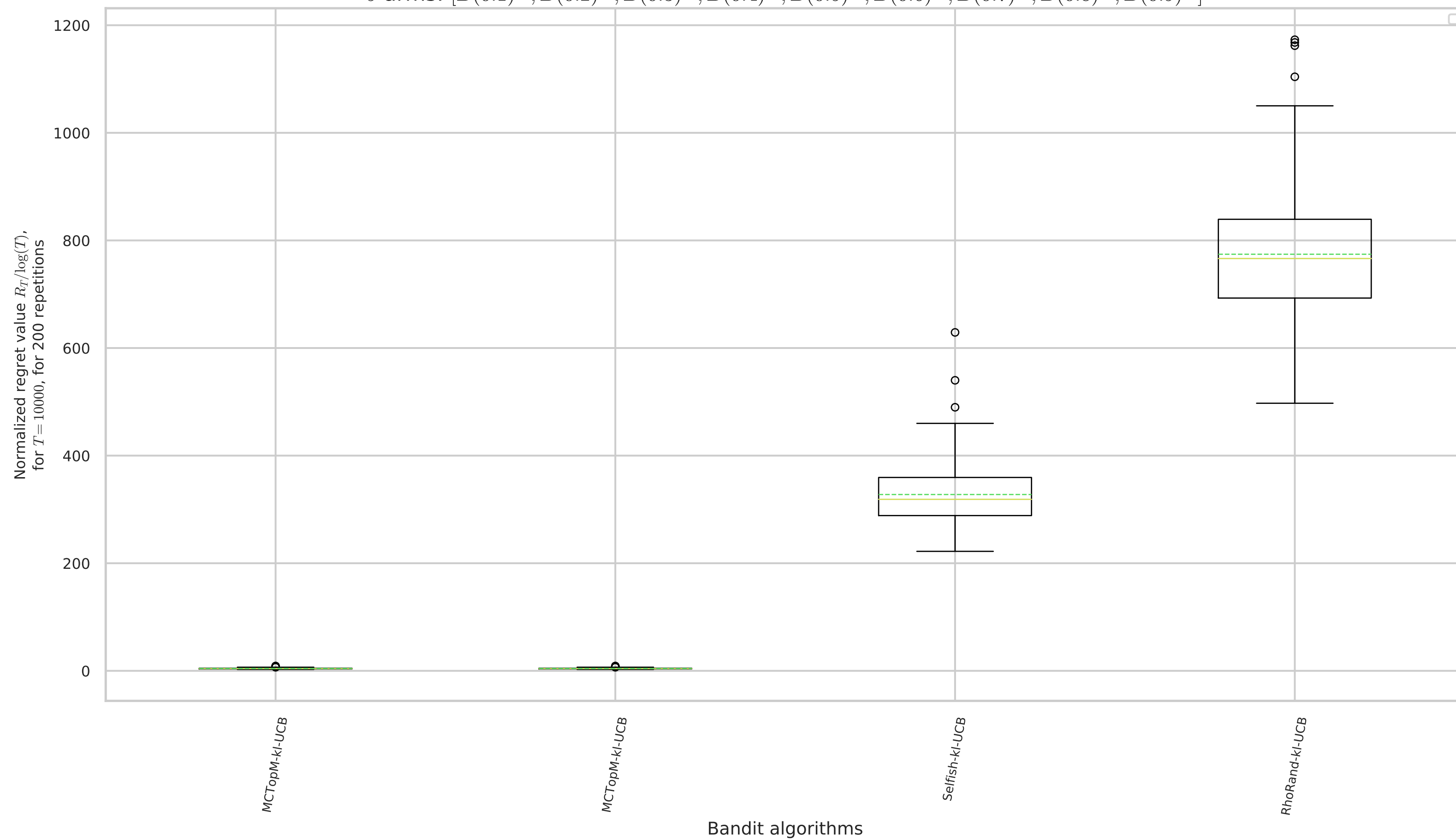
Multi-players M=9 : regrets for different bandit algorithms 9 arms: [B(0.1)^*, B(0.2)^*, B(0.3)^*, B(0.4)^*, B(0.5)^*, B(0.6)^*, B(0.7)^*, B(0.8)^*, B(0.9)^*]
