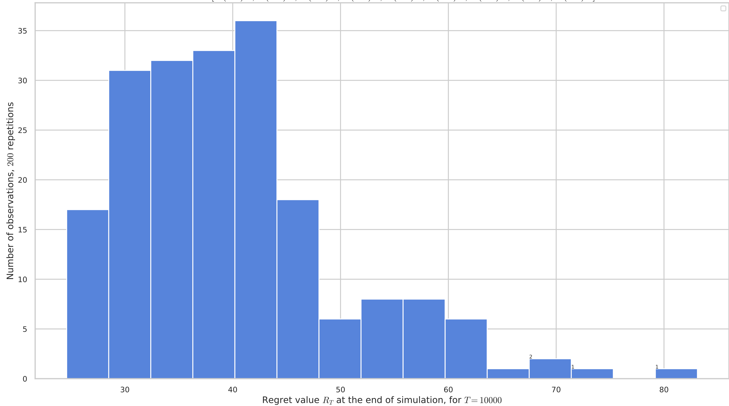
Multi-players M=9 : Histogram of regrets for MCTopM-kl-UCB 9 arms: [B(0.1)^*, B(0.2)^*, B(0.3)^*, B(0.4)^*, B(0.5)^*, B(0.6)^*, B(0.7)^*, B(0.8)^*, B(0.9)^*]
