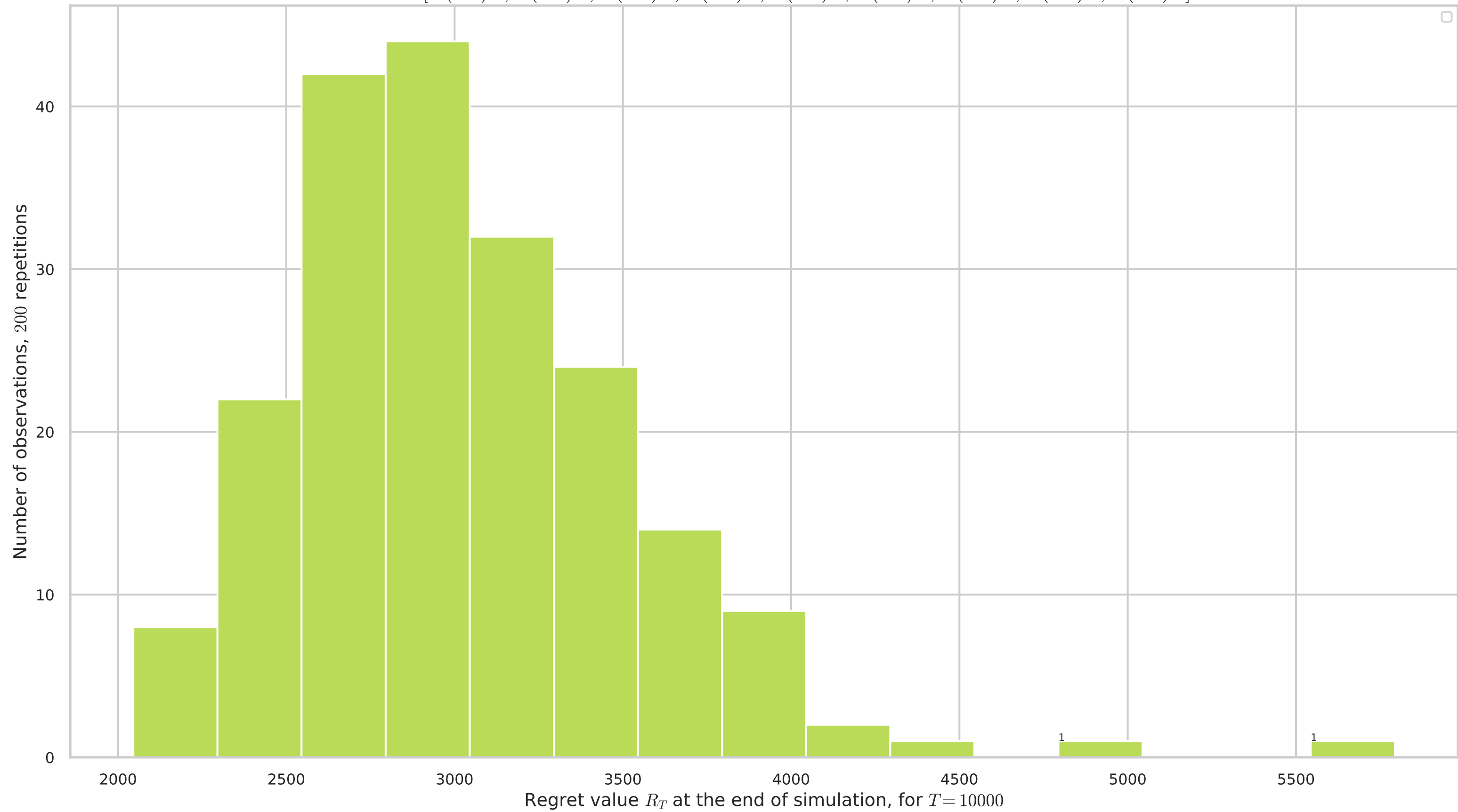
Multi-players M=9 : Histogram of regrets for Selfish-kl-UCB 9 arms: [B(0.1)^*, B(0.2)^*, B(0.3)^*, B(0.4)^*, B(0.5)^*, B(0.6)^*, B(0.7)^*, B(0.8)^*, B(0.9)^*]
