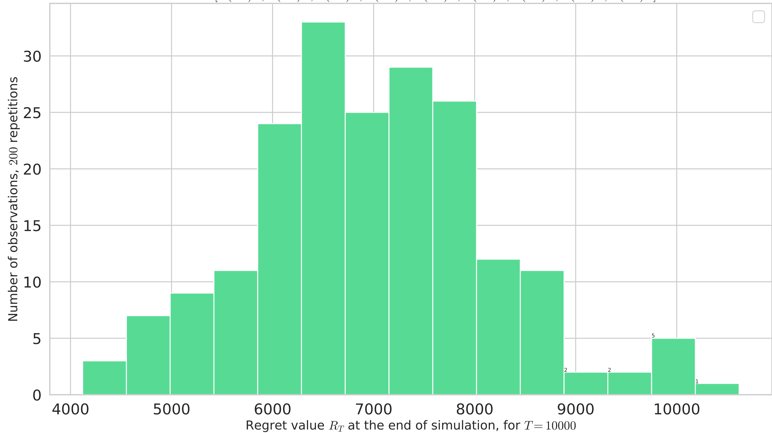
Multi-players M=9 : Histogram of regrets for RhoRand-kl-UCB 9 arms: [B(0.1)^*, B(0.2)^*, B(0.3)^*, B(0.4)^*, B(0.5)^*, B(0.6)^*, B(0.7)^*, B(0.8)^*, B(0.9)^*]
