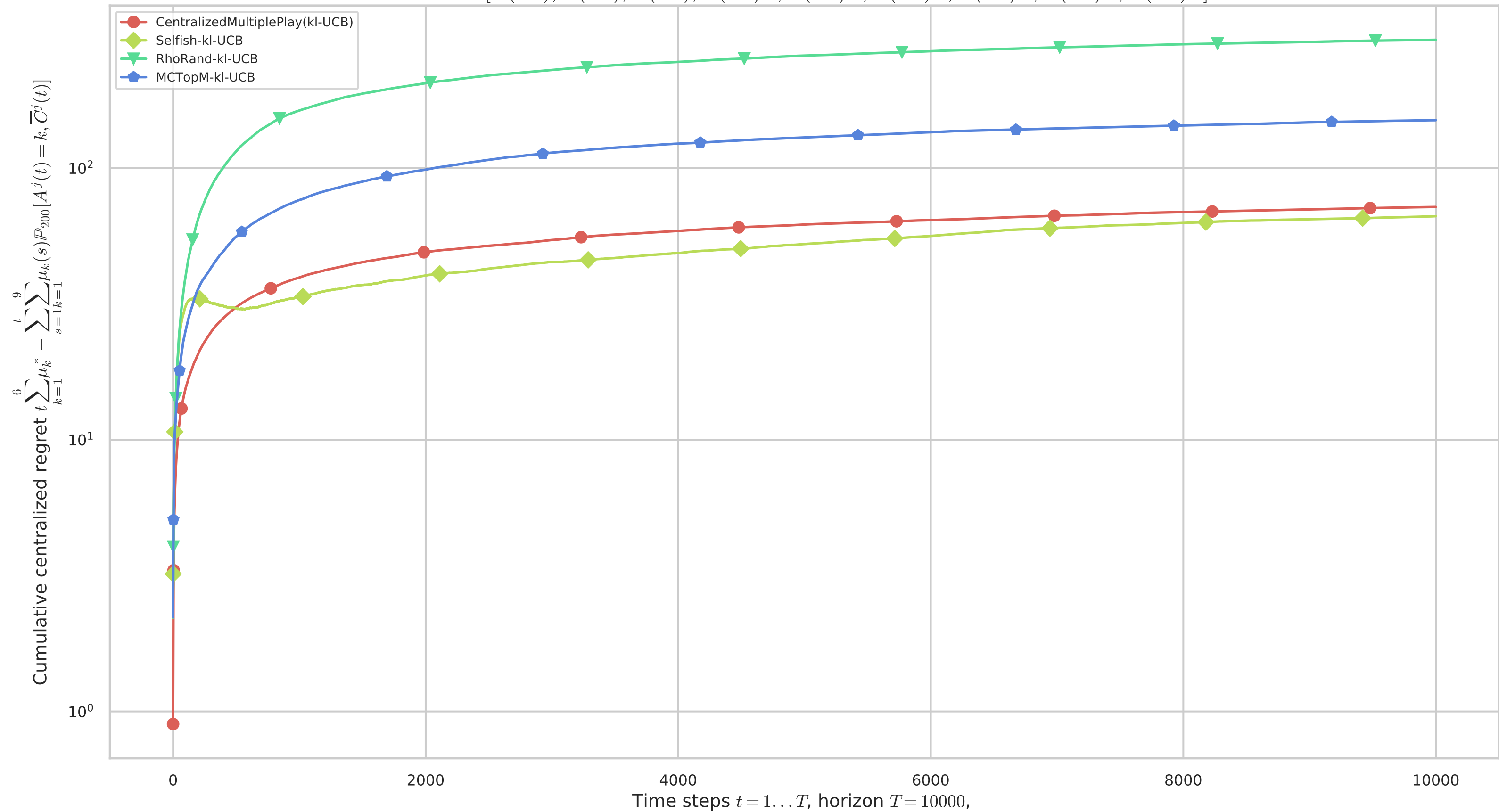
Multi-players M=6 : Cumulated centralized regret, averaged 200 times 9 arms: [B(0.1), B(0.2), B(0.3), B(0.4)^*, B(0.5)^*, B(0.6)^*, B(0.7)^*, B(0.8)^*, B(0.9)^*]
