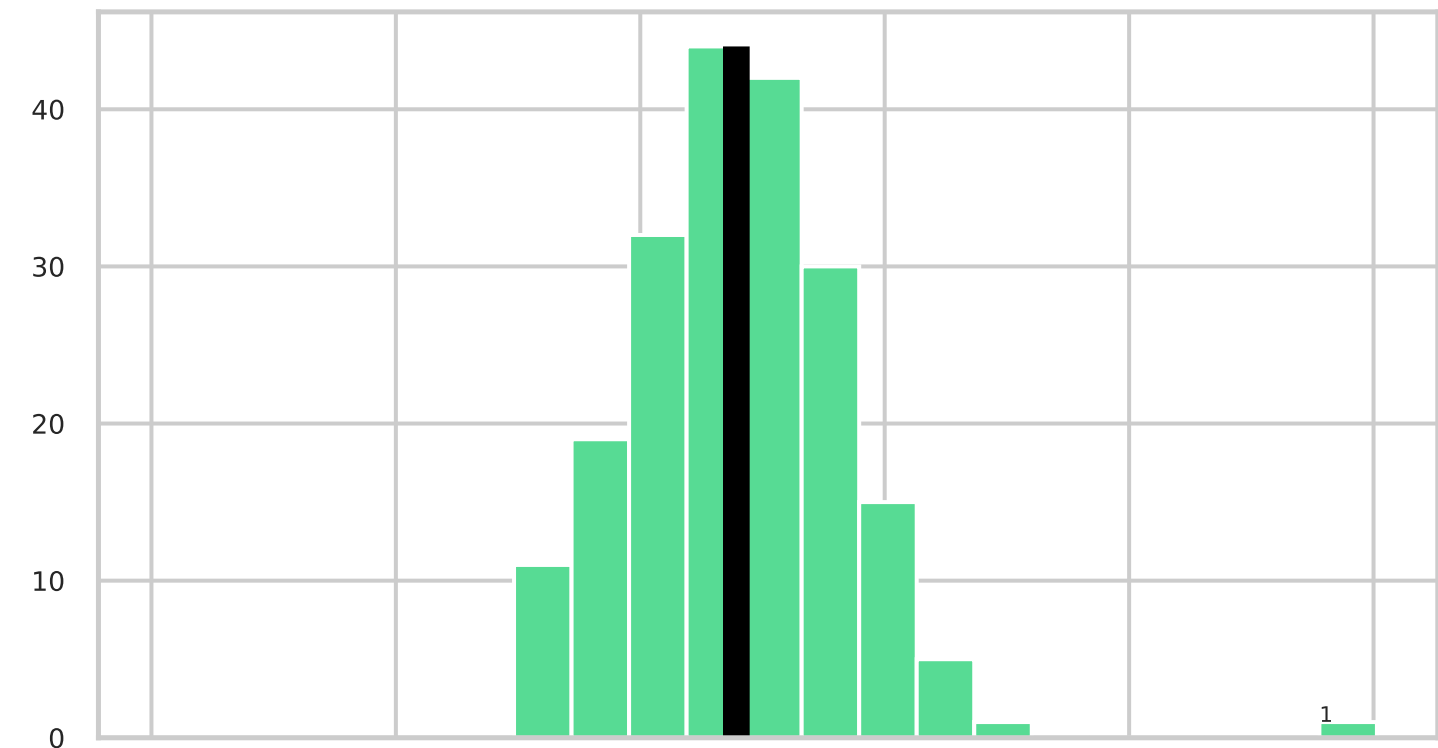
RhoRand-kl-UCB
