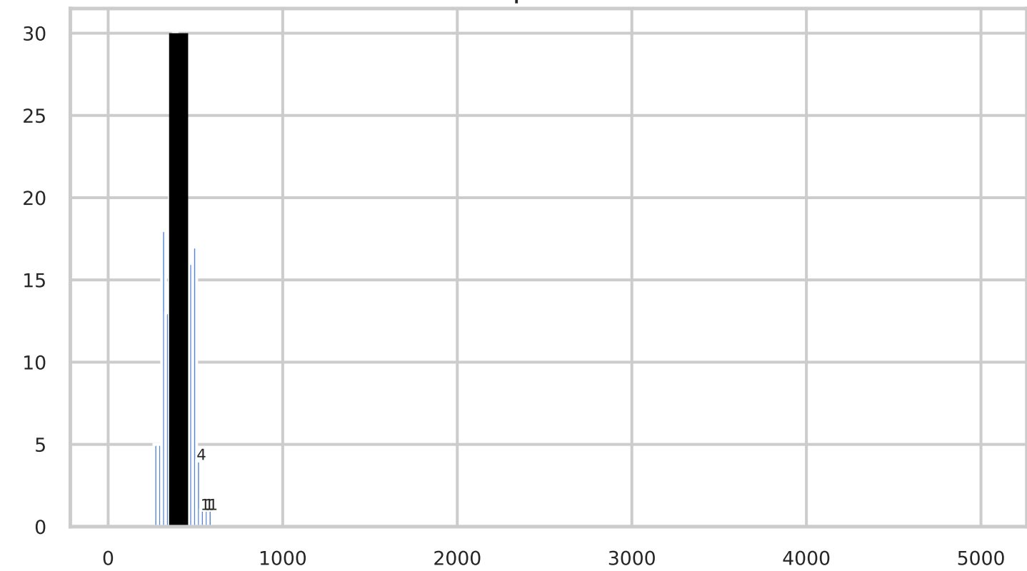
MCTopM-kl-UCB
