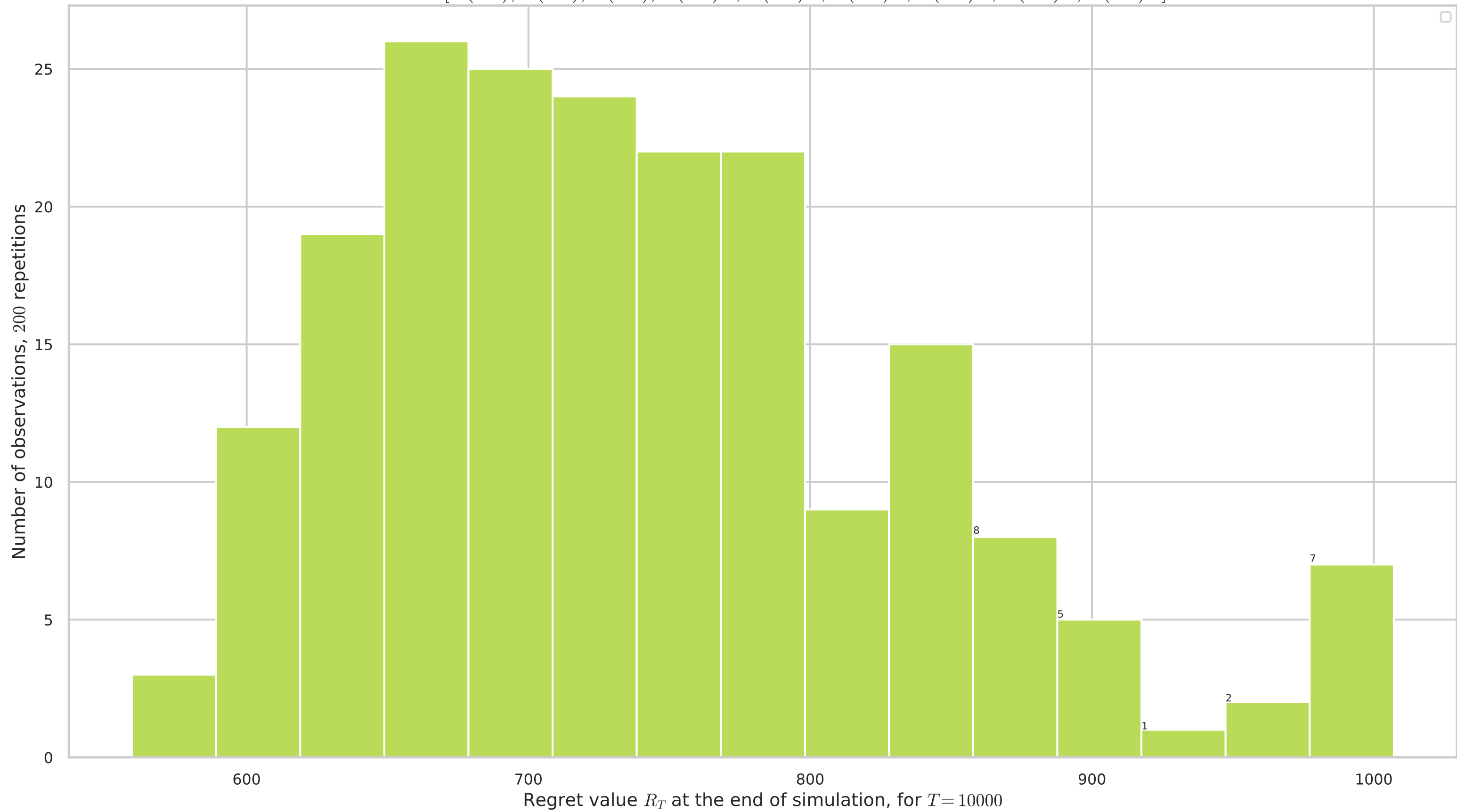
Multi-players M=6 : Histogram of regrets for Selfish-kl-UCB 9 arms: [B(0.1), B(0.2), B(0.3), B(0.4)^*, B(0.5)^*, B(0.6)^*, B(0.7)^*, B(0.8)^*, B(0.9)^*]
