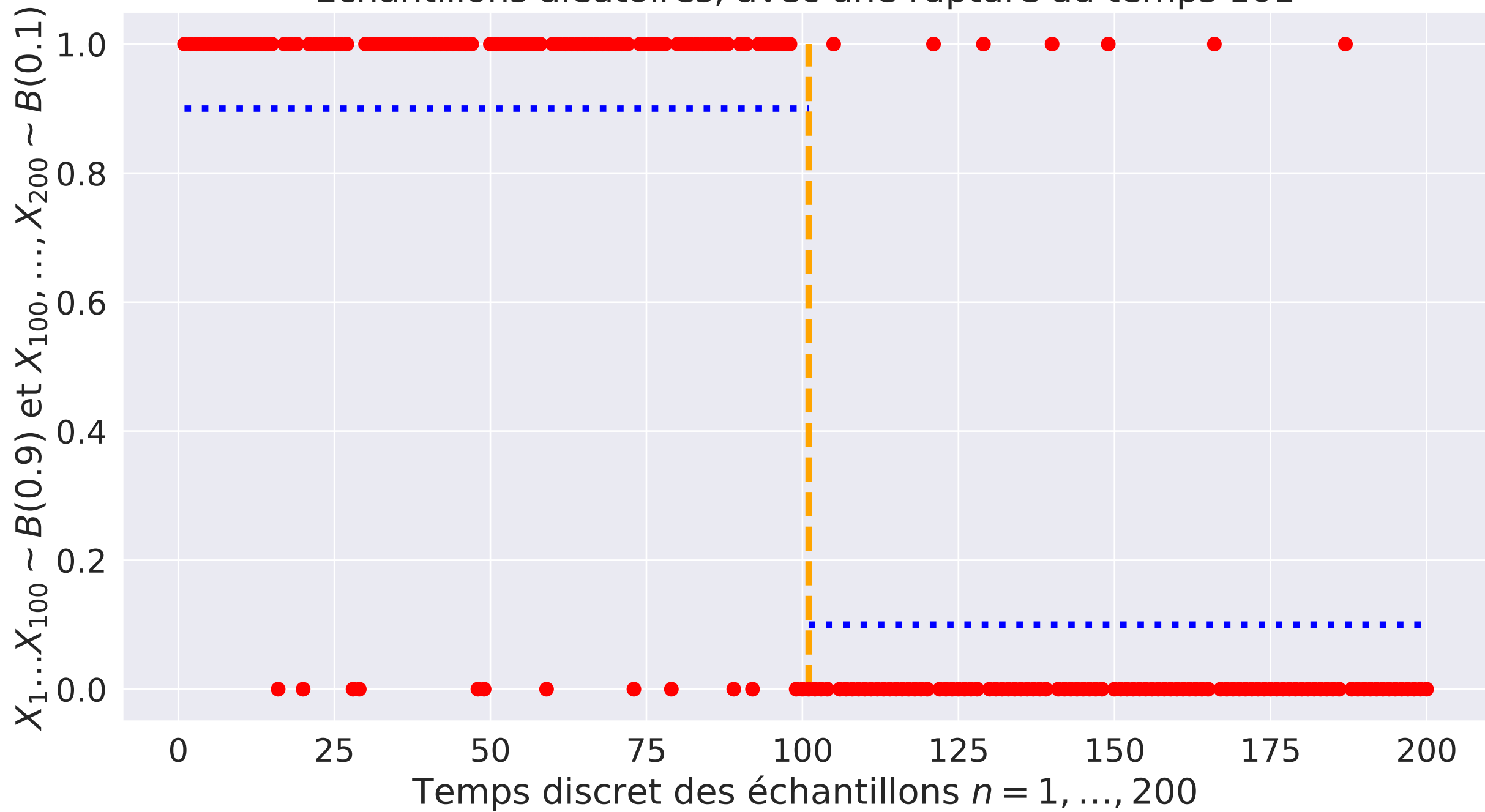
Échantillons aléatoires, avec une rupture au temps 101
