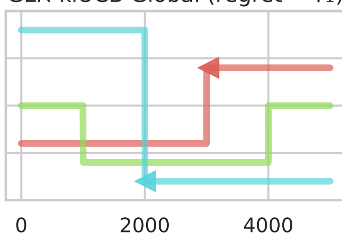
GLR-klUCB Global (regret = 71)
