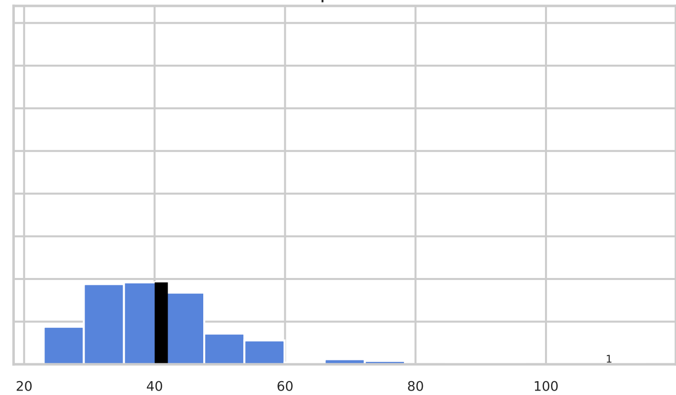
MCTopM-kl-UCB
