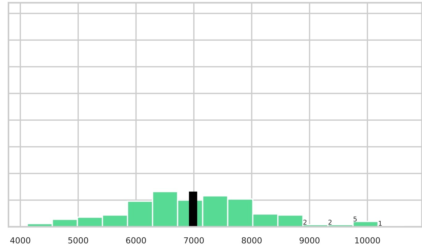
MCTopM-kl-UCB
