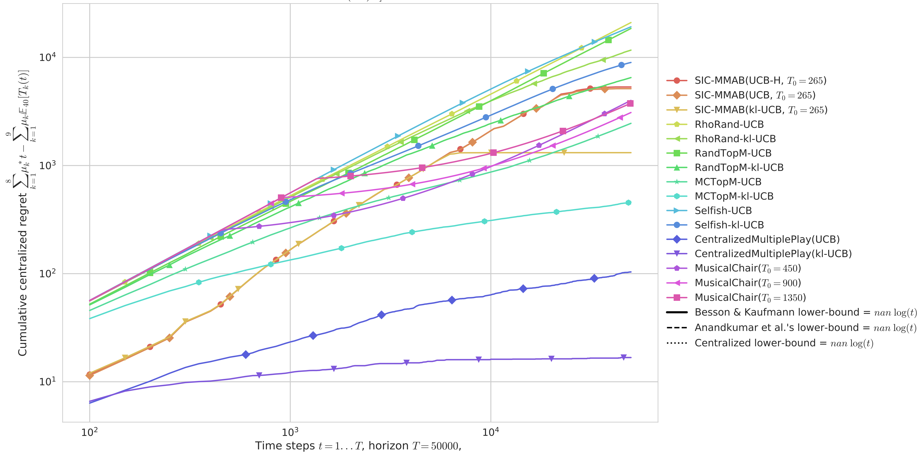
Multi-players M=8 : Cumulated centralized regret, averaged 40 times 9 arms: [B(0.01), B(0.01)^*, B(0.01)^*, B(0.1)^*, B(0.12)^*, B(0.14)^*, B(0.16)^*, B(0.18)^*, B(0.2)^*]
