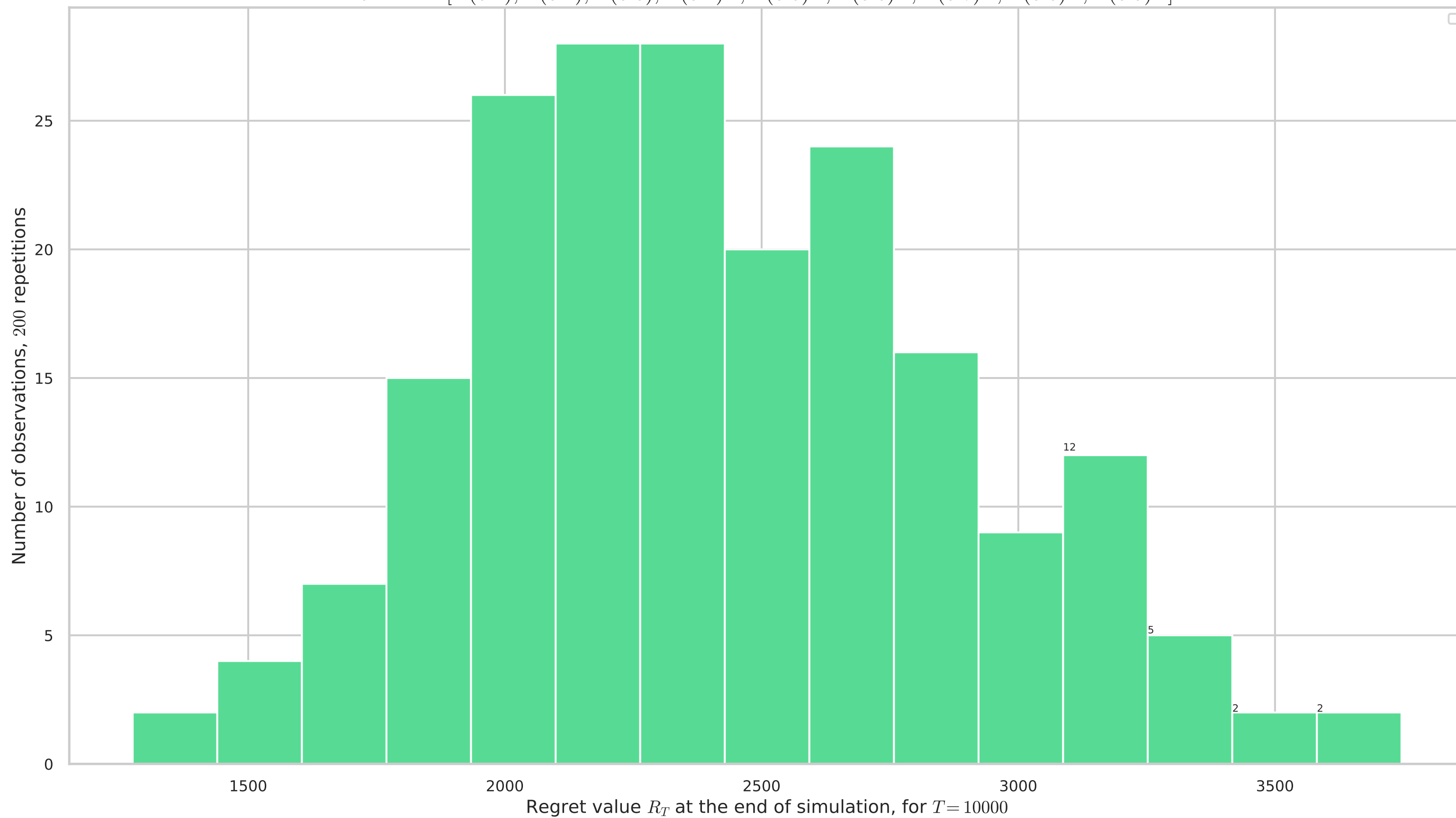
Multi-players M=6 : Histogram of regrets for RhoRand-kl-UCB 9 arms: [B(0.1), B(0.2), B(0.3), B(0.4)^*, B(0.5)^*, B(0.6)^*, B(0.7)^*, B(0.8)^*, B(0.9)^*]
