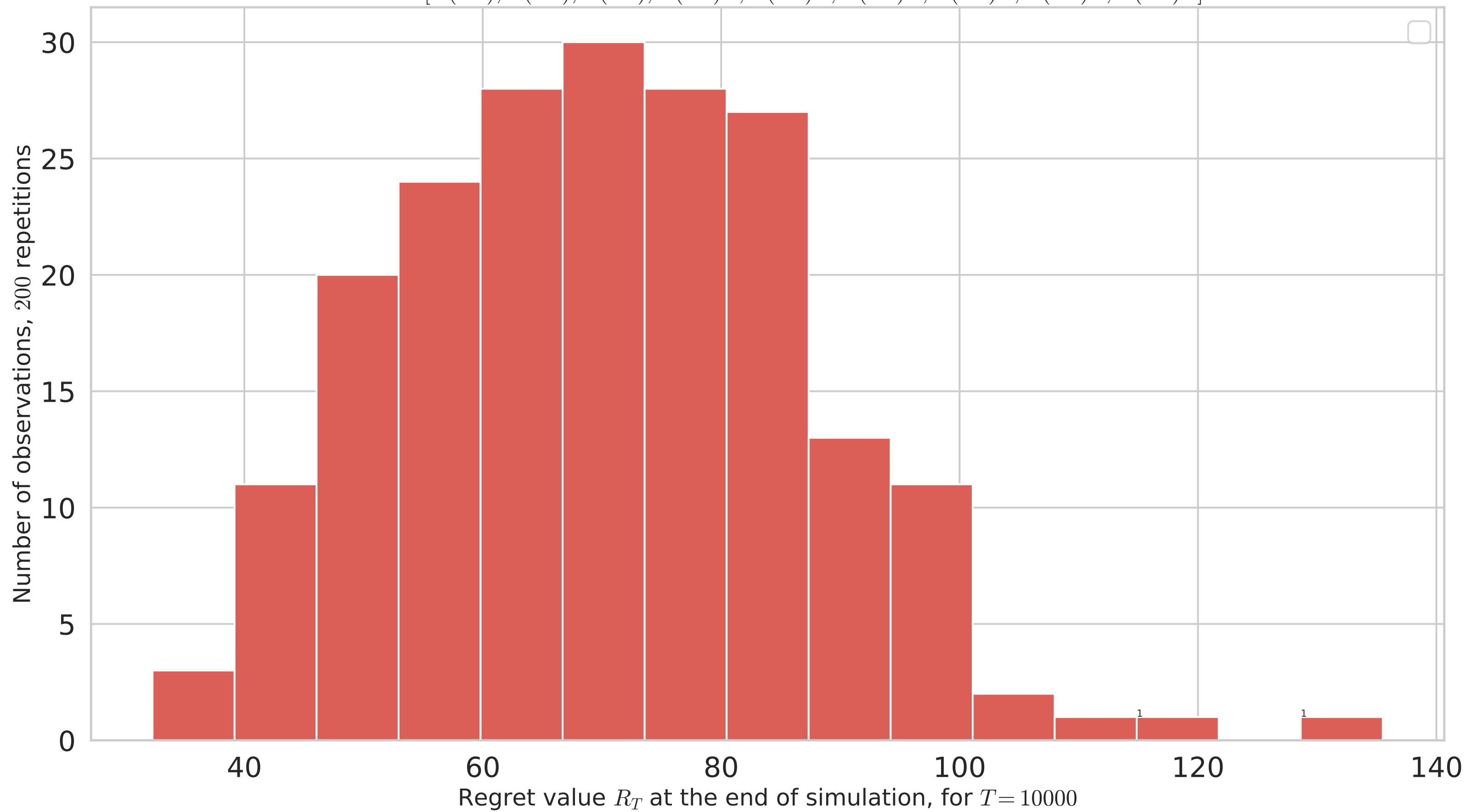
Multi-players M=6 : Histogram of regrets for CentralizedMultiplePlay(kl-UCB) 9 arms: [B(0.1), B(0.2), B(0.3), B(0.4)^*, B(0.5)^*, B(0.6)^*, B(0.7)^*, B(0.8)^*, B(0.9)^*]
