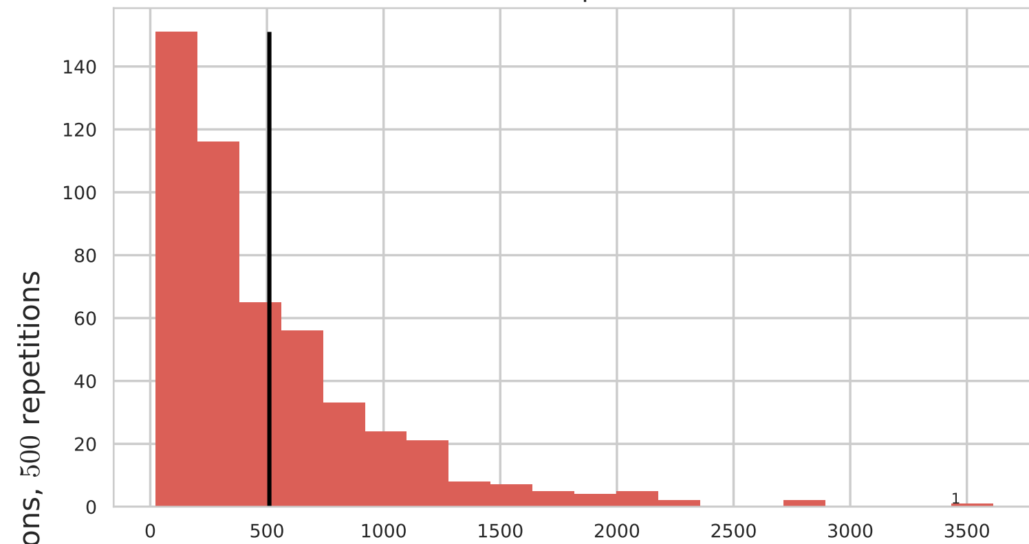
9 × MCTopM-KLUCB
