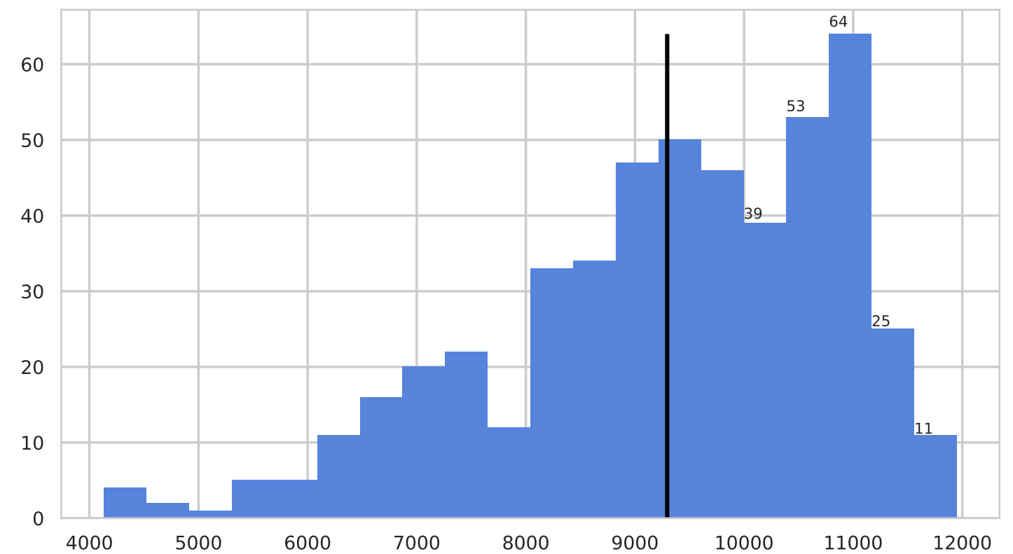
9 × RhoRand-KLUCB
