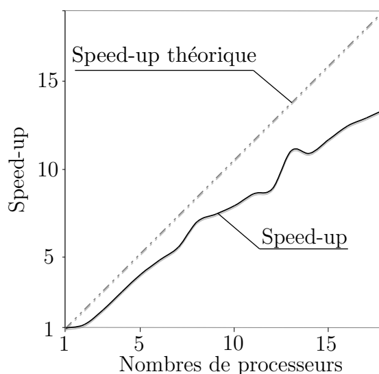
Figure 3.11: Speed-up pour le problème de la poutre.
