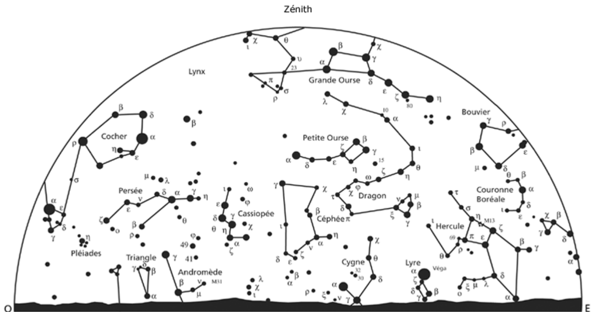
Aspects du ciel à Paris, image du haut vers le nord, image du bas vers le sud, le 1er avril vers 21 h 15 m UT ou le 16 vers 20 h 15 m UT.
