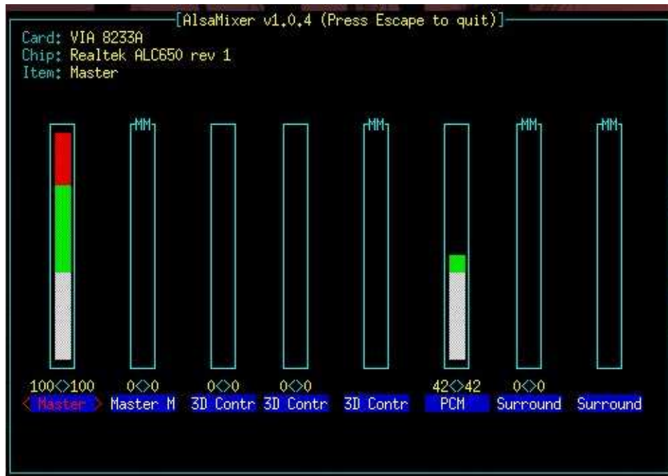
FIG. 3.1 – Alsamixer
