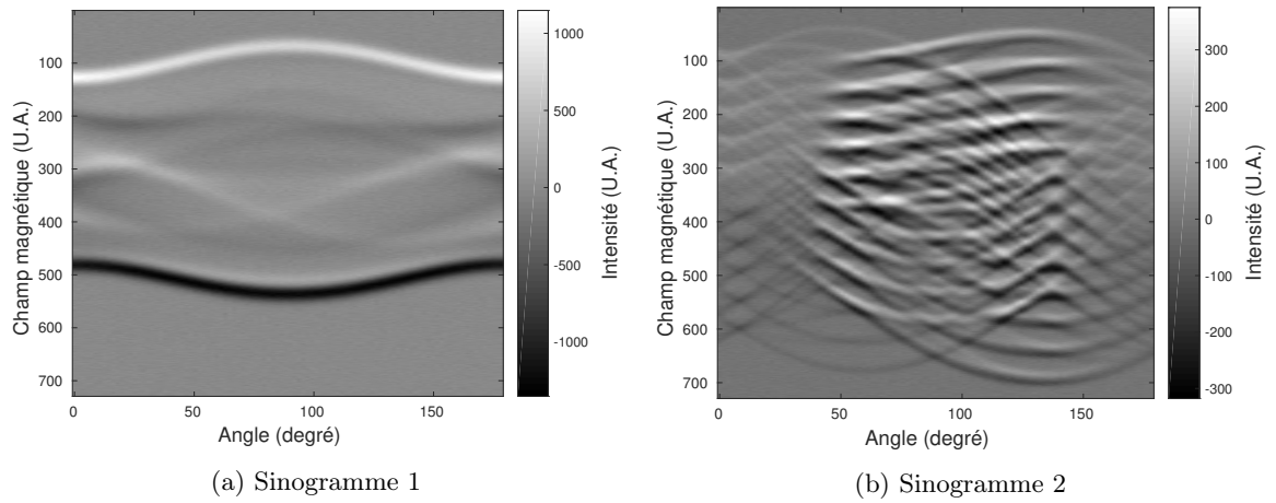
FIGURE 73 – Sinogrammes intermédiaires
