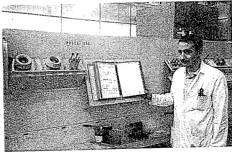
Fig. 3-12 - Usine Solex d'Evreux. Fiches d'instructions pour la préparation des outils de coupe destinés à un centre d'usinage. L'ensemble est situé à quelques mètres de la machine. Le constructeur de la machine effectue lui-même le pré-réglage de ses outils.
