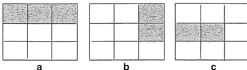
Fig. 9-5 - Trois exemples de matrices incomplètes.
