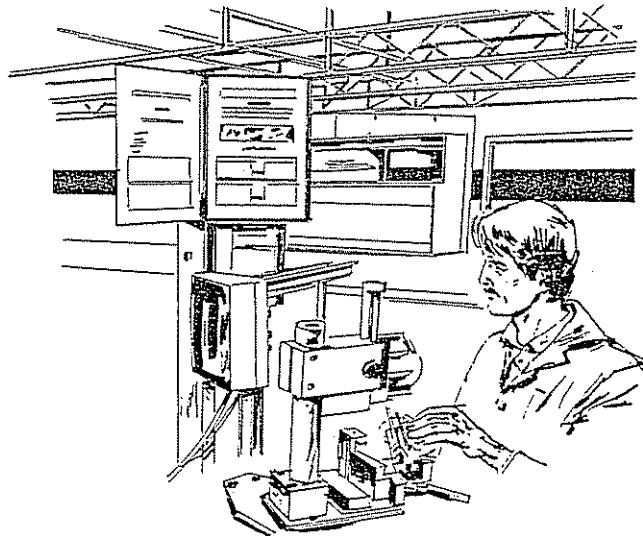
Fig. 3-2 - Documentation visuelle. Les fiches d'instructions sont présentes près du poste de travail (voir détail fig. 3-14).
