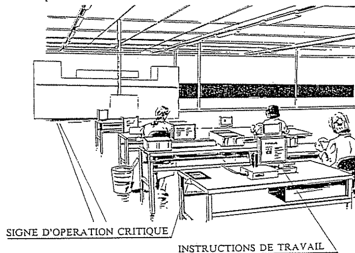
Fig. 3-7 - Usine Siemens de Toulouse. Comme les documents sont trop nombreux pour être laissés à demeure près du poste, des supports en U ont été installés pour recevoir les fiches amovibles glissées entre deux plaques transparentes. On notera également la présence sur le coin gauche de certaines tables d'une plaque qui indique que l'opération est critique pour la qualité finale du produit. Ce type de signe est un exemple intéressant de documentation visuelle. Il se voit bien (la couleur est jaune) et son emploi évite de surcharger une fiche d'instructions.
