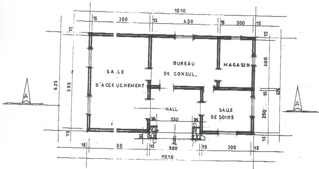
Vue en plan ech=1:100
